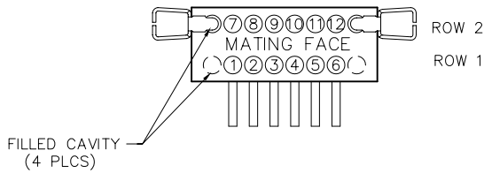
PLUG MA-2B1-012-325-A5200
