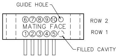
PLUG MA-251-010-325-A6600
