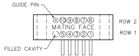
RECEPTACLE MA-261-010-435-A6300
