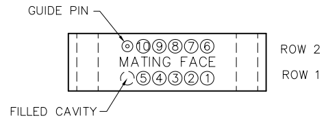
RECEPTACLE MA-221-010-261-A63WA
